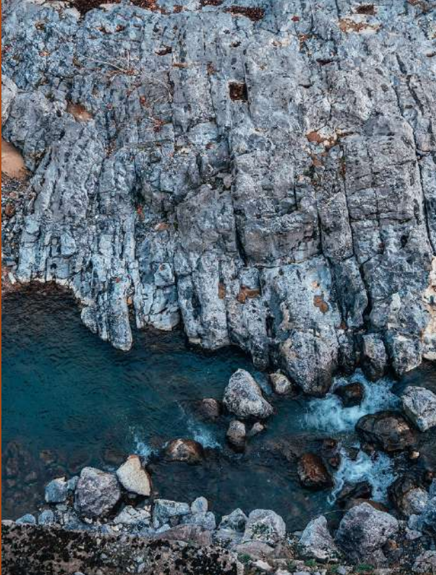
Gökgöl Devoniyen Karbonifer Sınır İstifi
